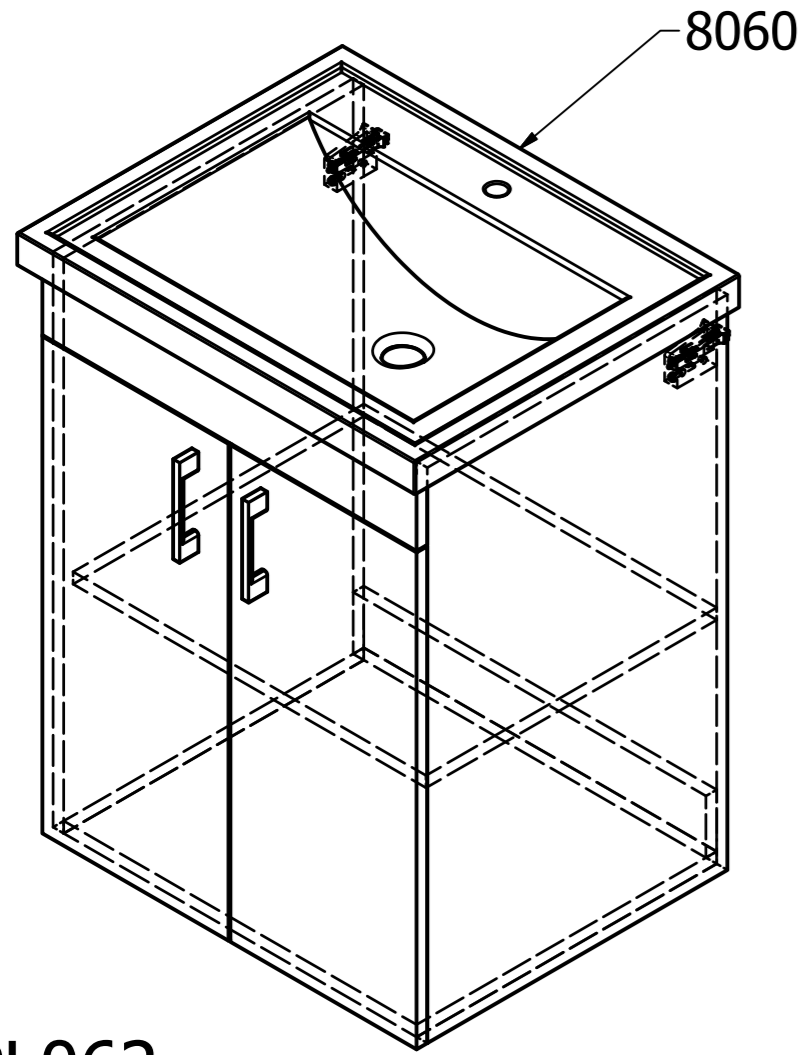
PL062 560x746x465 - skříň 595x780x485 - celek
