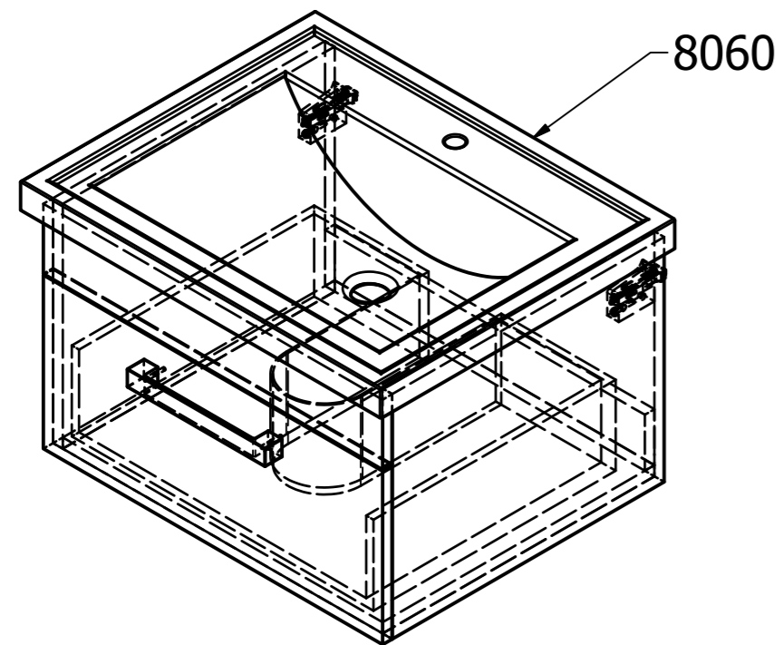
57081 560x350x465 - skříň 595x384x485 - celek
