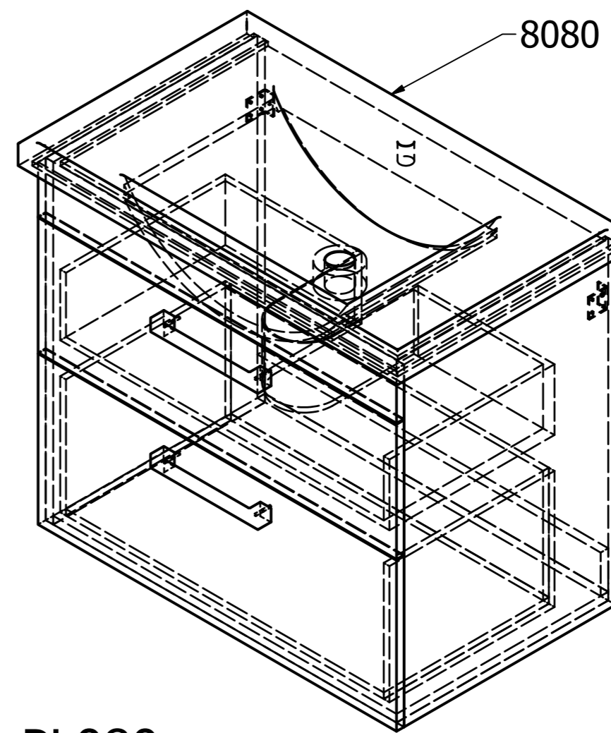
PL080 760x666x465 - skříň 805x700x485 - celek
