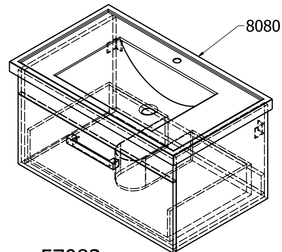
57083 760x400x465 - skříň 805x434x485 - celek
