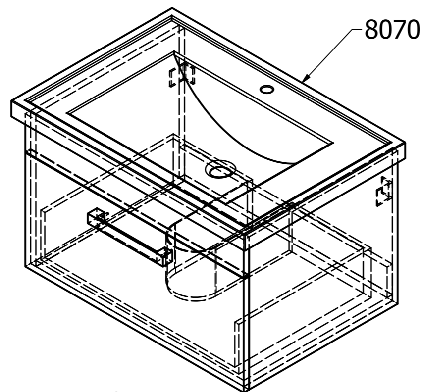
57086 660x400x465 - skříň 705x434x485 - celek
