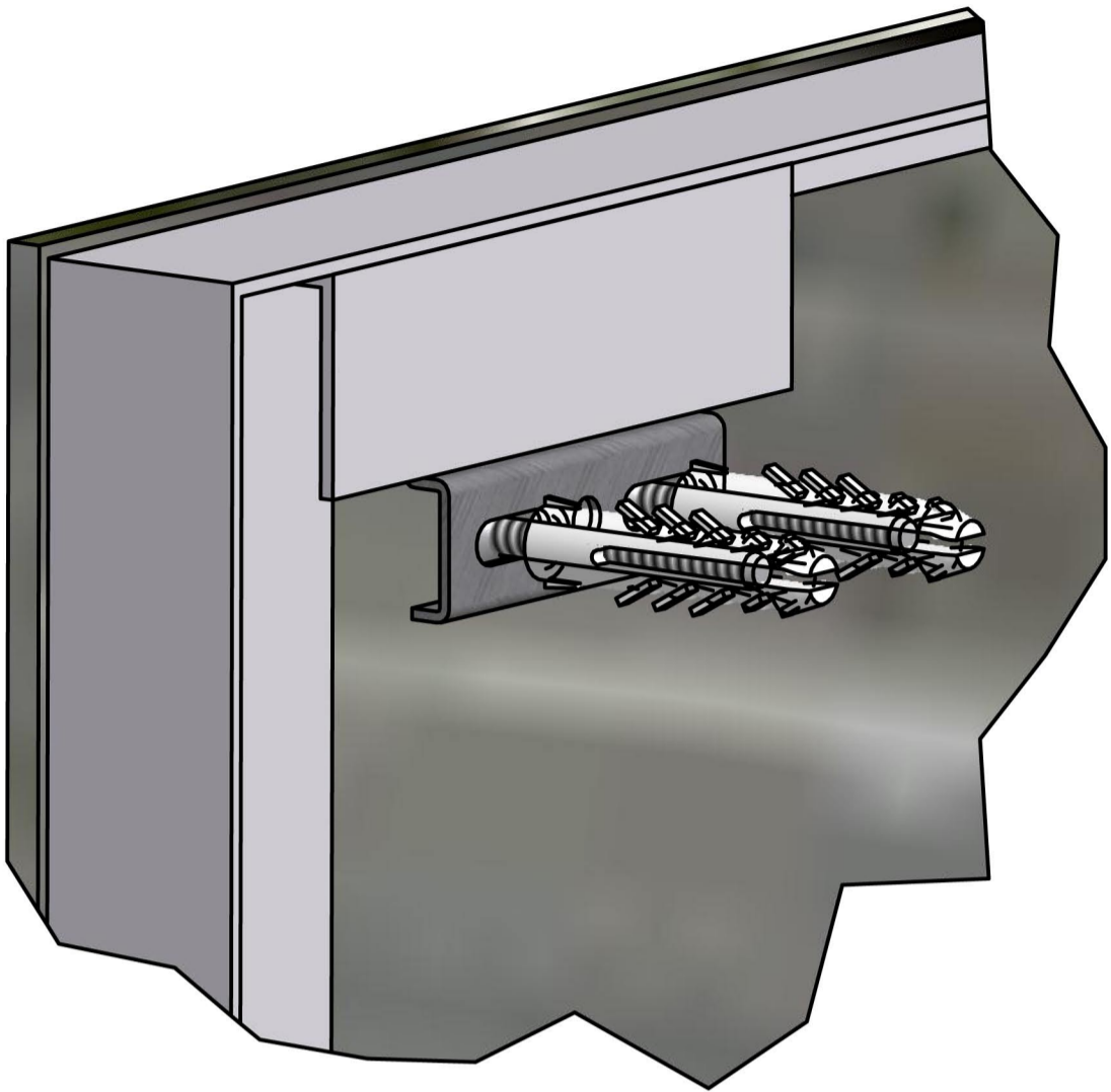
DETAIL PŘIDĚLÁNÍ DO ZDI
