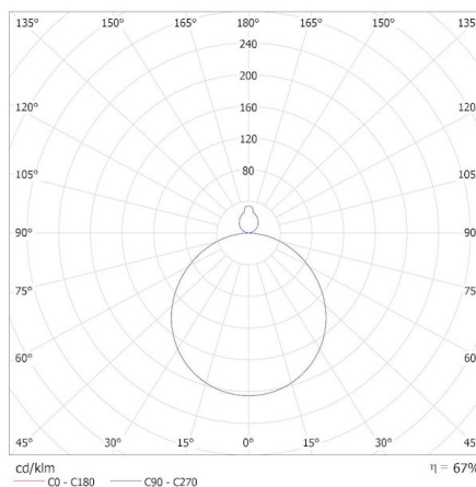
MILED0 (kat 31502) AZPO LED 18,5W-NW-O-W / Krzywa rozsytu światła (biegunowo)
