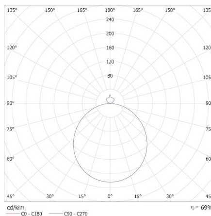
MILED o (kat 31500) AZPO LED 11,8W-NW-O-W / Krzywa rozsyłu światła (biegunowo)
