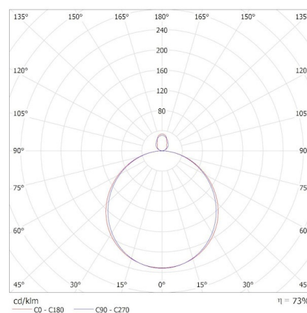
MILED o (kat 31511) AZPO LED 22W-NW-L-B / Krzywa rozsyłu światła (biegunowo)
